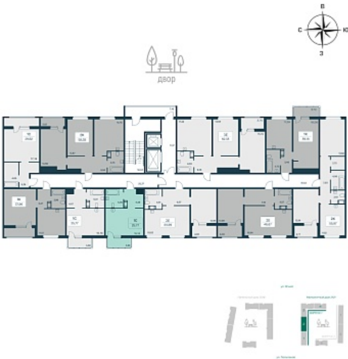
План этажа
